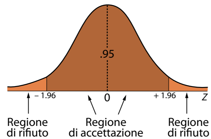
GRAFICO 1. CURVA NORMALE STANDARD, CON EVIDENZIATA LA REGIONE DI RIFIUTO, CON \alpha = 5\%
